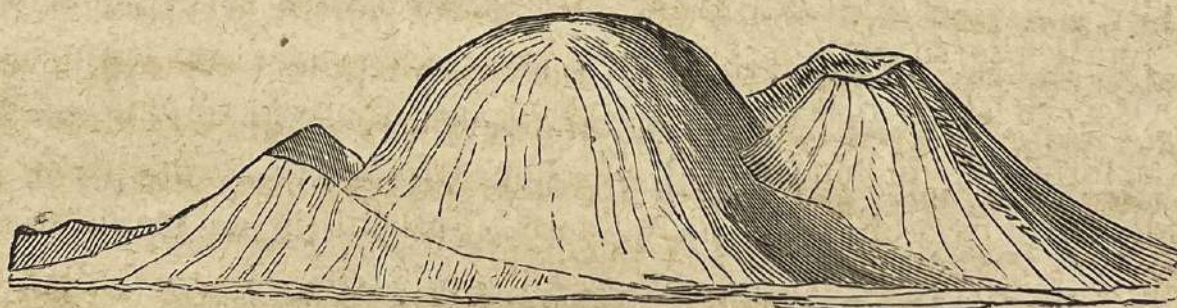
Fig. 8. — Puy di Sarcouy ; domo trachitico sorgente tra il Puy-de-la-Goutte e il piccolo Sarcouy , coni di ceneri nell'Alvernia.
