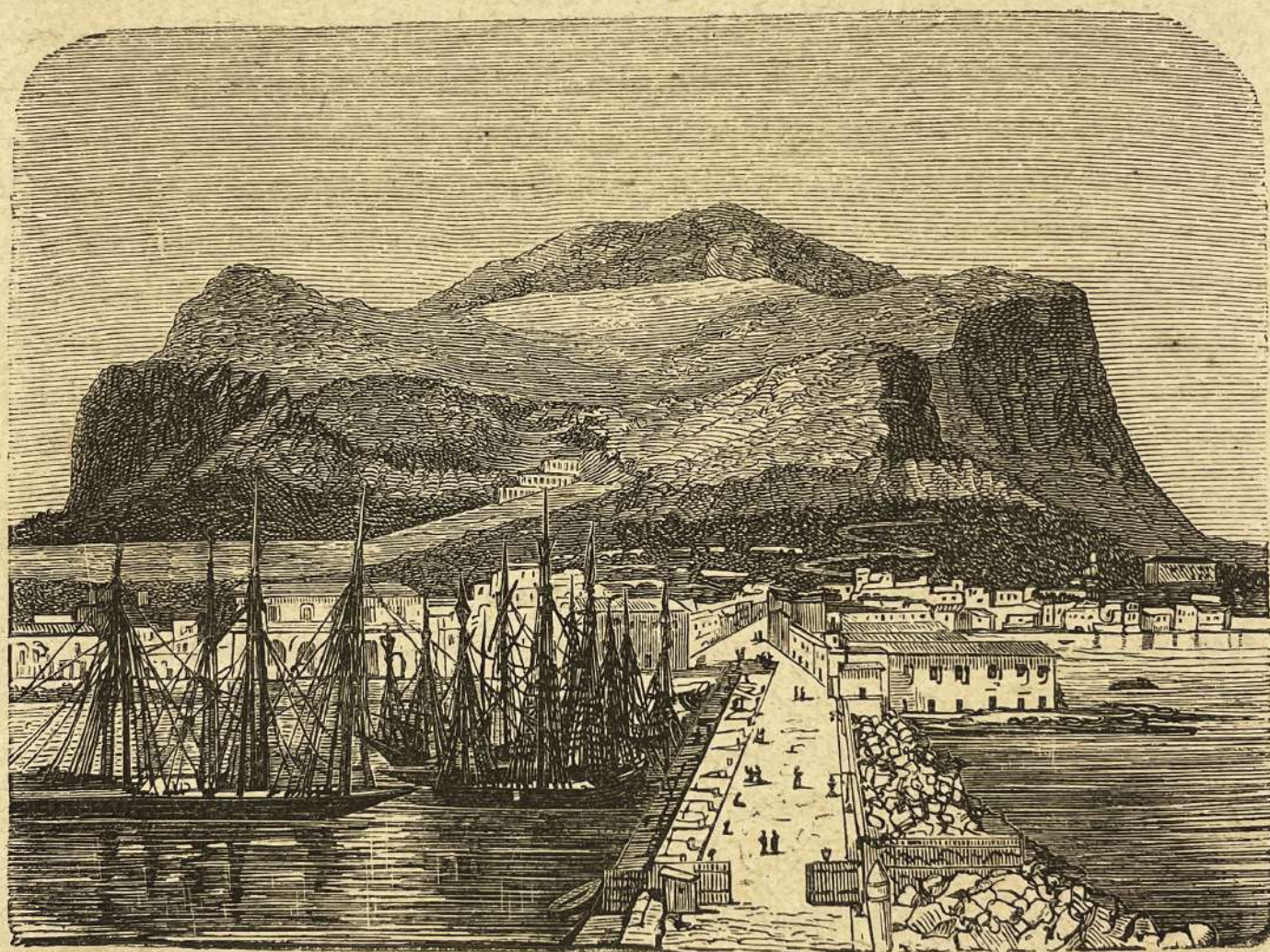
Fig. 32. — Veduta del Monte Pellegrino a Palermo.
