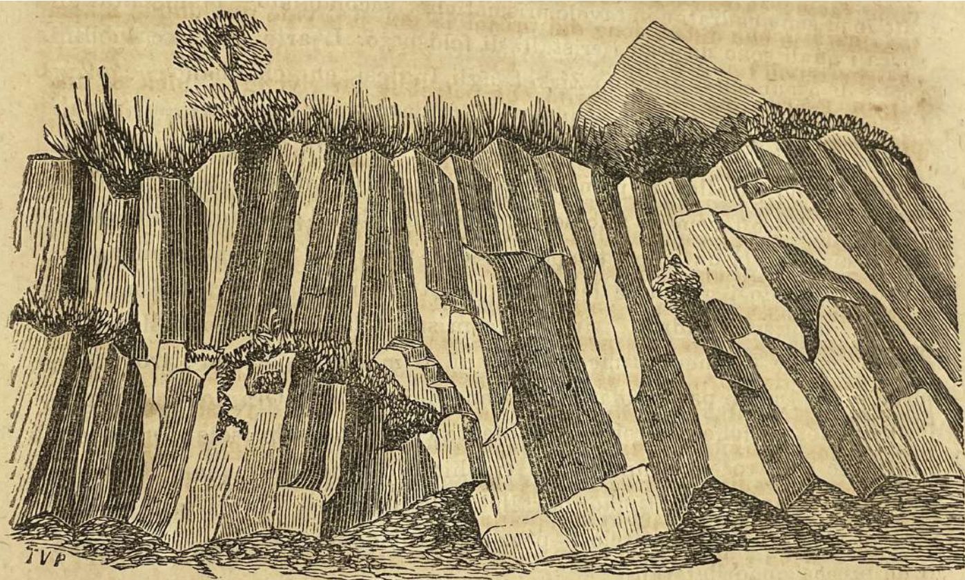
Fig. 52. — Colonnato di porfido sul lago di Lugano.
